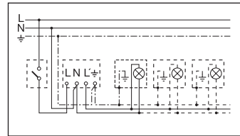
1. Valaisimet ilman nolajohtinta
