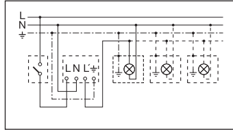
2. Lámpara con conductor neutro implantado
