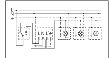
4. Koppling via 2-polig brytare för fast sken respektive automatisk
