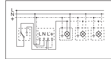
4. Liitäntä vaihtokytkimen välityksellä jatkuvaa valaistusta automaattikäyttöä varten
