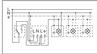
4. Tilkopling via vendebryter for kontinuerlig lys og automatisk drift
