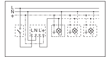
2. Belysning med befintlig nolldare
