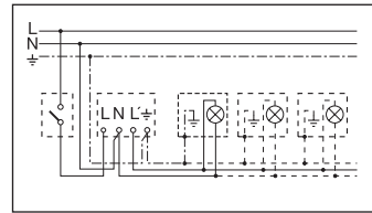
1. Belysning utan nolldare
