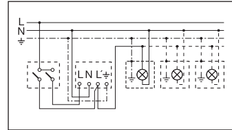
3. Liitäntä sarjakytkimen välityksellä käsi- ja automaattikäyttöön
